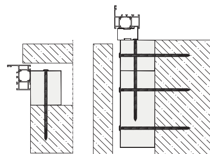
seitliche Ansicht Stütze
