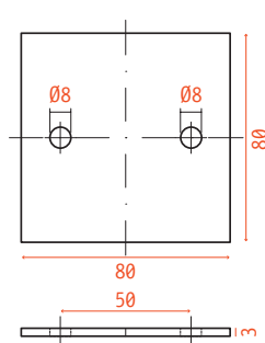
Befestigungsplatte
