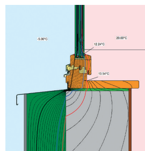
Herkömmliche Montage: Fenster in der Mauerlaibung
